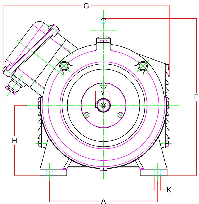
Motori a corrente continua "AP" serie pesante Esecuzione IP23 protetta contro lo stitlicidio, autoventilata DC "AP" (open with feet) motors - heavy line IP23 execution protected against tripping, self-ventilated
